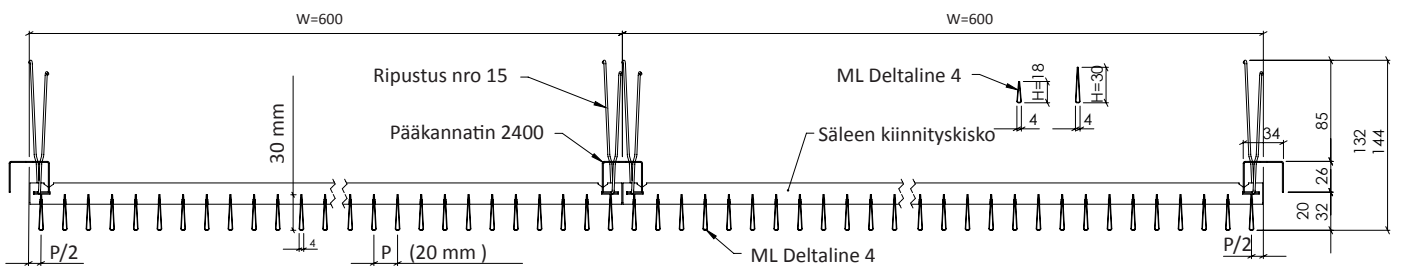
2 Ripustinjousi Nro 15
