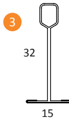
Pääkannatin 3700 nro 14
