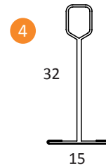
Välilista 1200 nro 15
