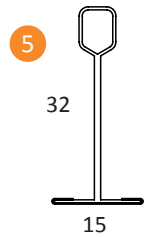
Välilista 600 nro 16
