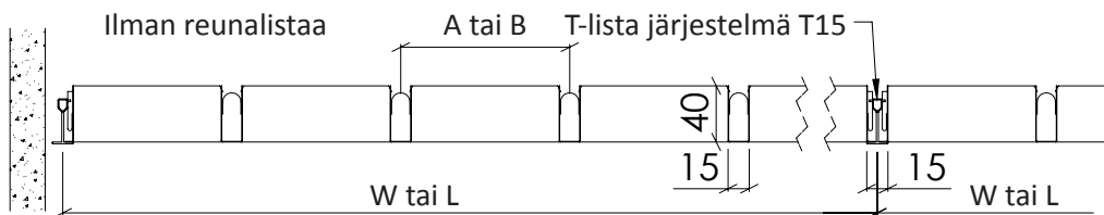
Pääkannatin 3700 nro 14
